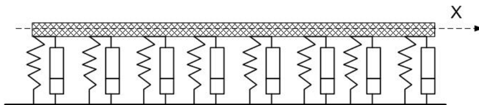
Рисунок Д.3 – Модель отброшенной части основания
