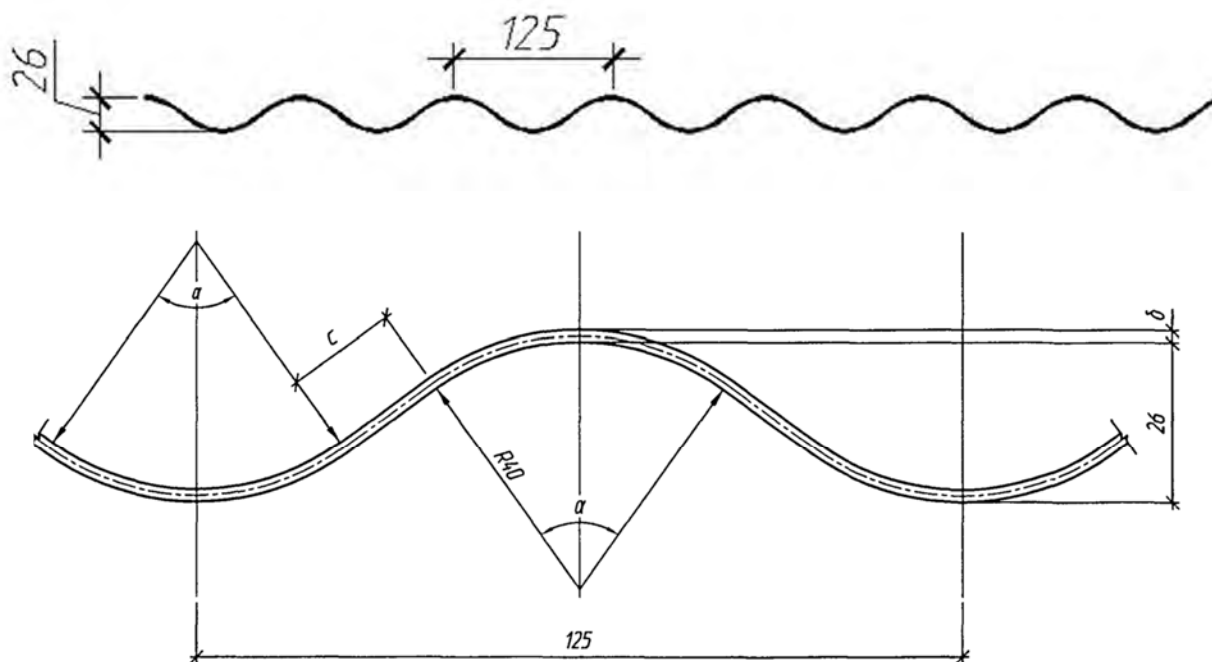
Рисунок А.2 – Параметры гофра 125x26
