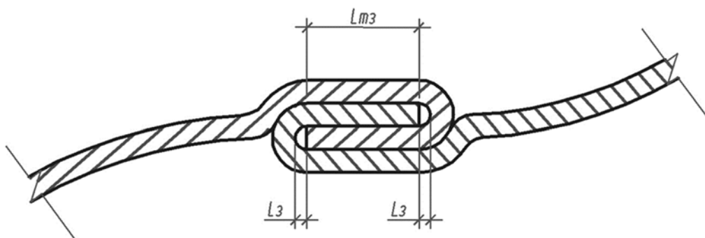
Рисунок 2 – Замковое соединение
