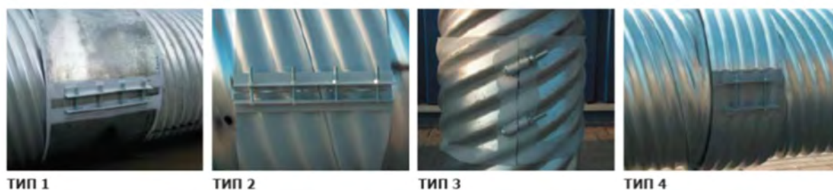
Рисунок А.8 – Внешний вид бандажных соединений СВМГТ
