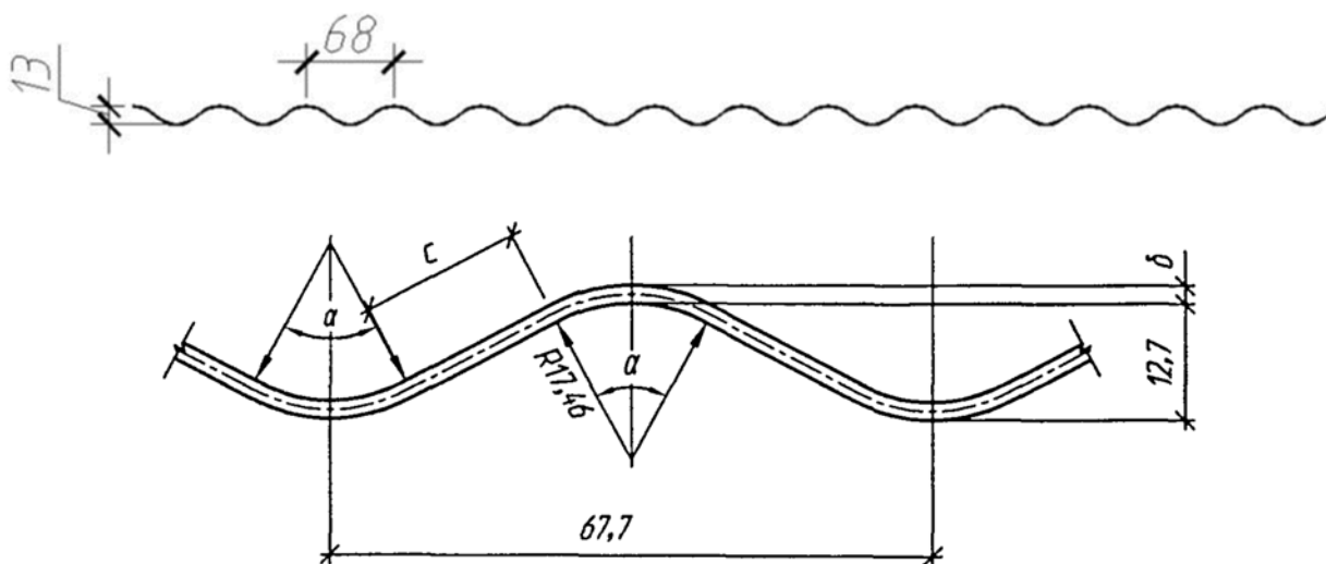
Рисунок А.1 – Параметры гофра 68x13
