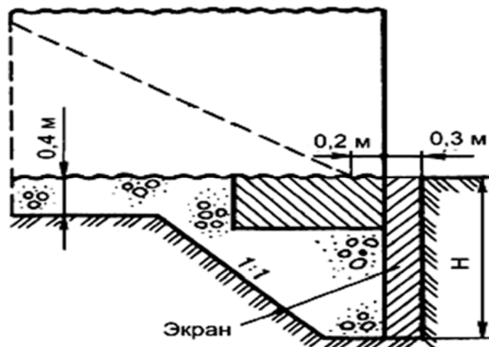
Рисунок 8 – Бетонный противофильтрационный экран
