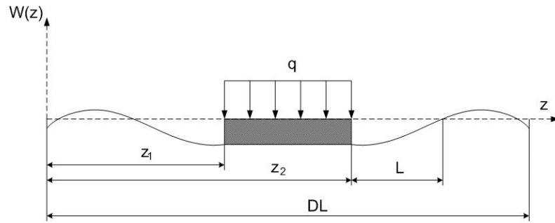
Рисунок Д.5 – Деформация основания от приложенной нагрузки
