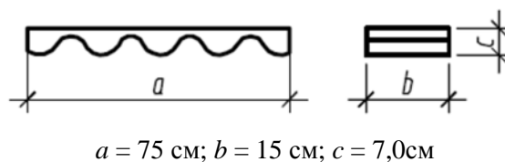
Рисунок Л.3 – Блок сборного лотка СВМГТ, гофр 150x50 мм
