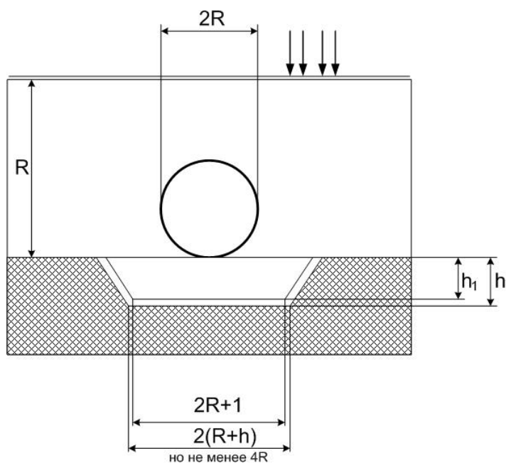
Рисунок Д.1 – Фрагмент системы, моделируемой по МКЭ
