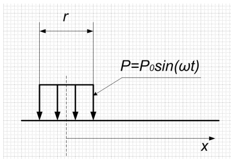
Рисунок Д.8 – Схема динамического нагружения основания
