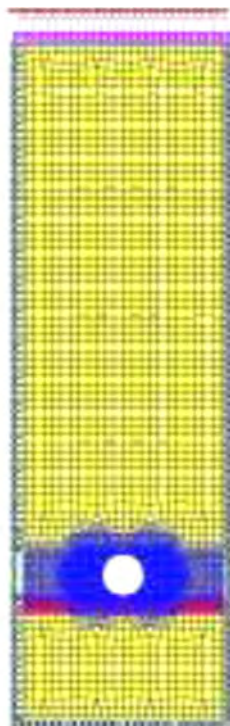
Рисунок Ж.1 – Конечно-элементная расчётная модель трубы, работающей совместно с грунтом засыпки ( D = 1,0 м, H = 12 м, \psi = 233 кН/м, автомобильная нагрузка НК14) Число узлов – 5575, число элементов – 5668, в том числе балочных – 124, элементов плоской деформации – 5544
