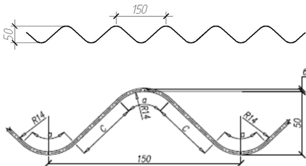
Рисунок А.3 – Параметры гофра 150x50
