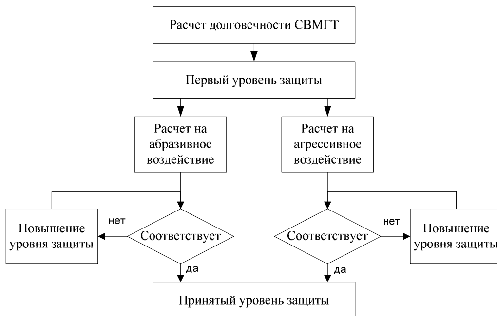
Рисунок 5 – Алгоритм прогнозирования долговечности СВМГТ
