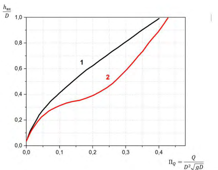
Рисунок И.1 – График для определения глубины потока на входе в СВМГТ
